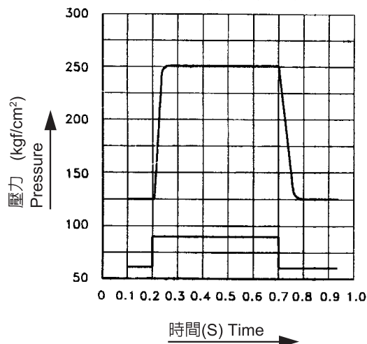
應答特性 Response Function ER - G01 - 3 - 10
