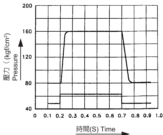
應答特性 Response Function ER - G01 - 2 - 10
